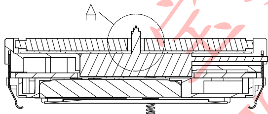
A-A 配AL21石英机芯
