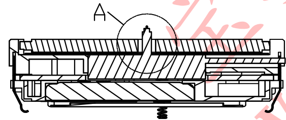
A-A 配AL21石英机芯
